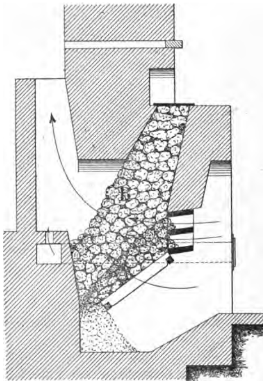
Fig. 66. — Foyer à décrassage continu.
